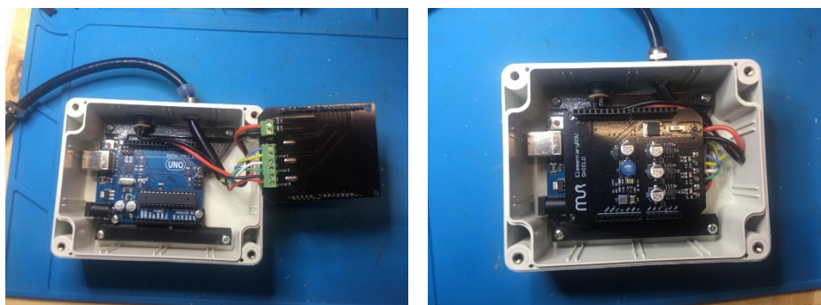
Рис. 10. Подключение моторов
